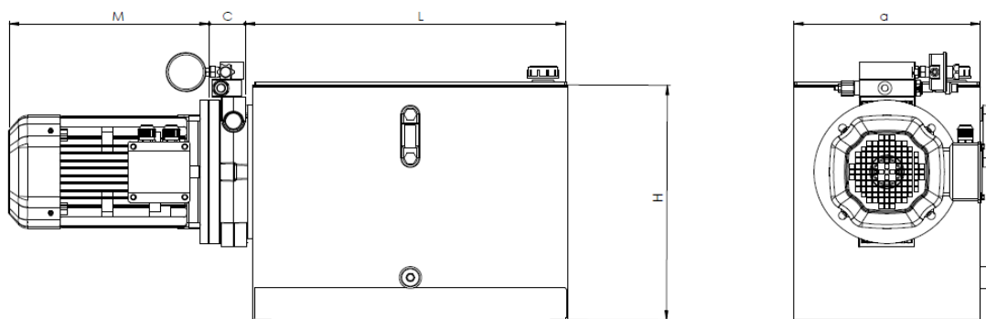
Montaje Horizontal
