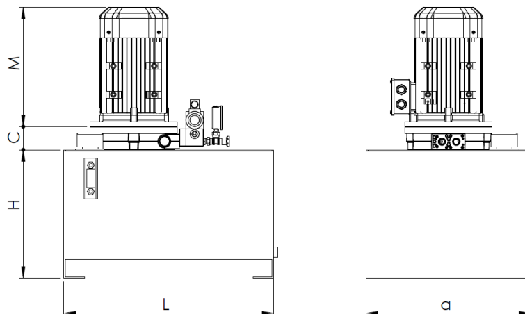
Montaje Vertical
